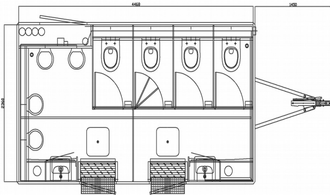
Toilettenwagen Typ2 4 Toiletten 4 Urinale
